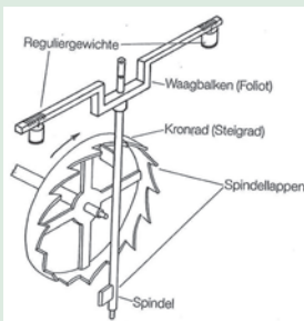
Waagbalkenhemmung
